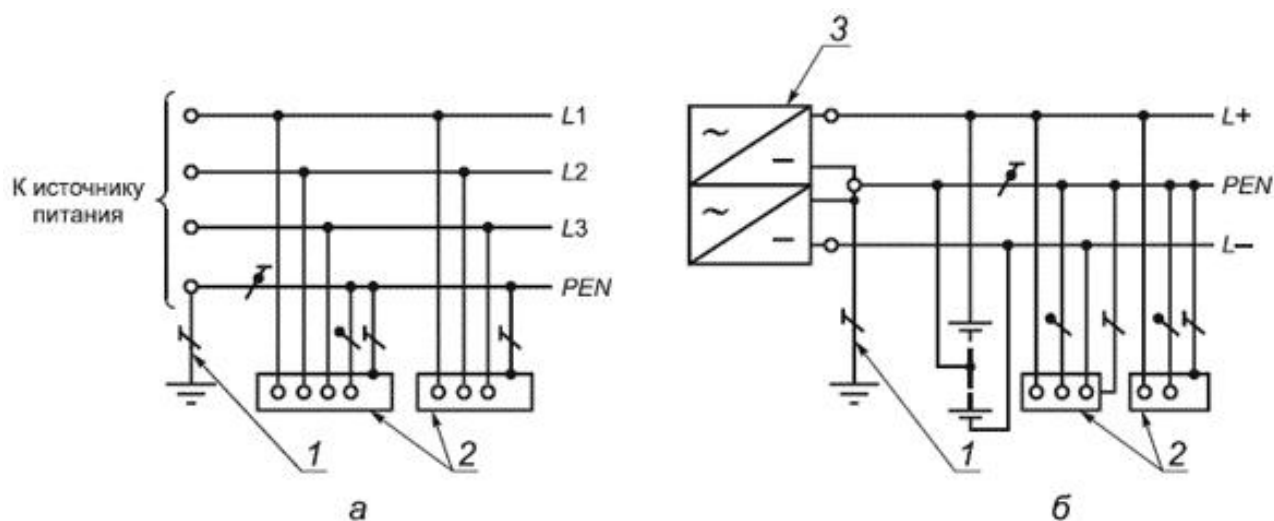
Рисунок 6 - Система TN-C переменного и постоянного тока
