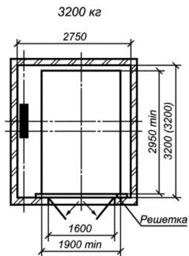
Высота кабины 2200. Высота дверного проема 2200
