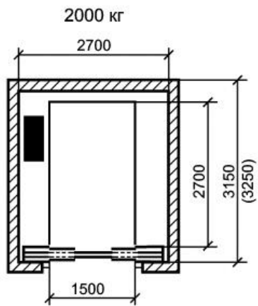
2000 кг Высота кабины 2100. Высота дверного проема 2100
