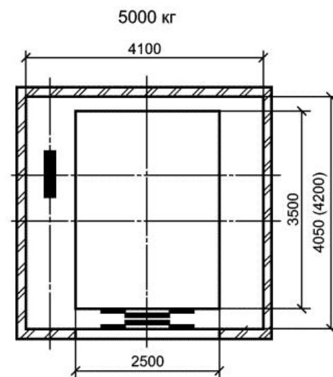
Высота кабины 2500. Высота дверного проема 2500
