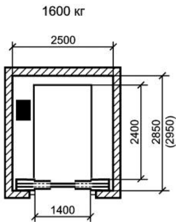
1600 кг Высота кабины 2100. Высота дверного проема 2100
