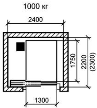
1000 кг Высота кабины 2100. Высота дверного проема 2100
