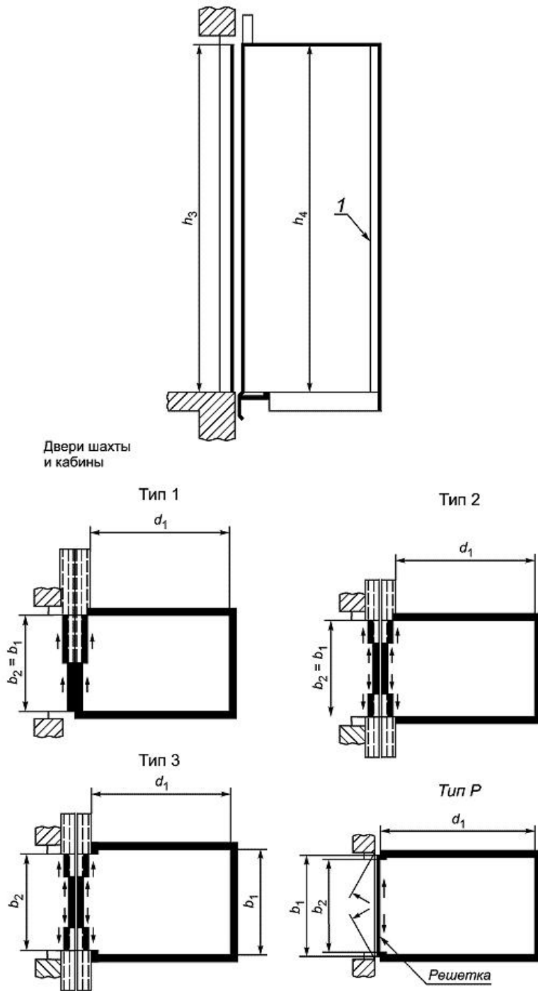
Рисунок 1 - Грузовые лифты. Обозначения размеров кабины и дверного проема, лист 1,2
