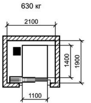
630 кг Высота кабины 2100. Высота дверного проема 2100
